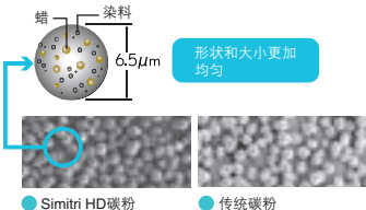
Simitri HD碳粉的结构
